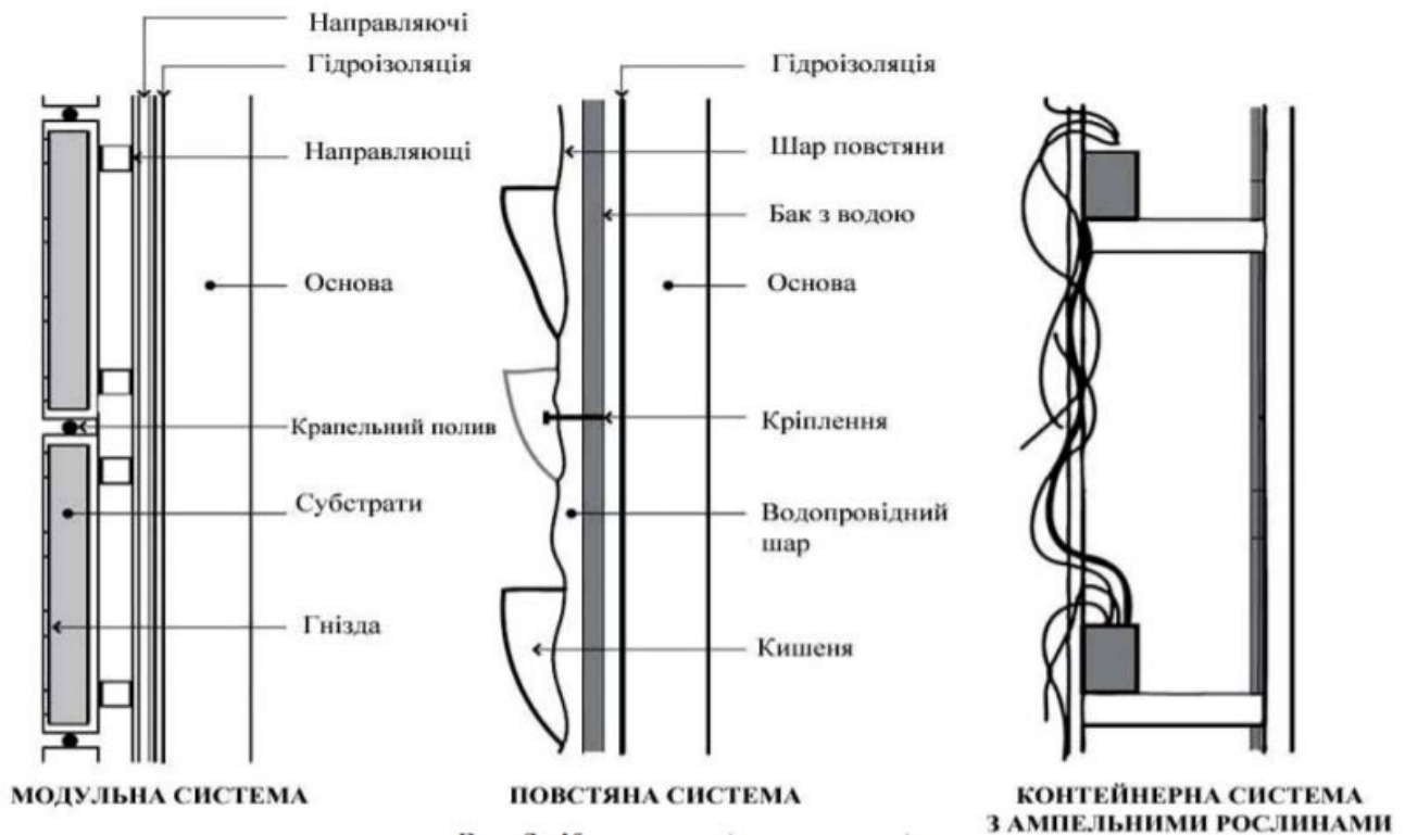
Рис.4. Схеми систем вертикального озеленення
